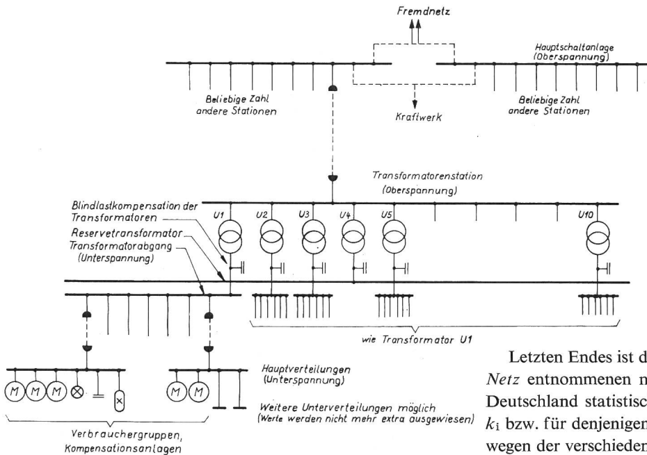
Fig. 2 Vereinfachtes Übersichtsschema für das untersuchte Energieversorgungsnetz [72]
