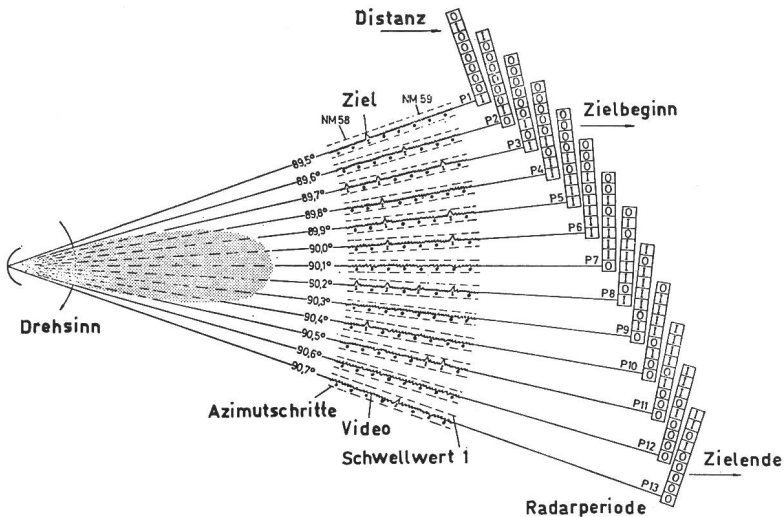
Fig. 11 Prinzip des Gleitfensterdetektors Die digitalisierten Echoimpulse werden einem Schieberegister zugeführt, dessen kumulierter Inhalt ein Mass für die Lagewahrscheinlichkeit des Zielschwerpunktes darstellt P zeitliche Folge der Radarimpulse
