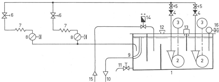
Fig. 11 Schema des Stehlagers-Kühlsystems
