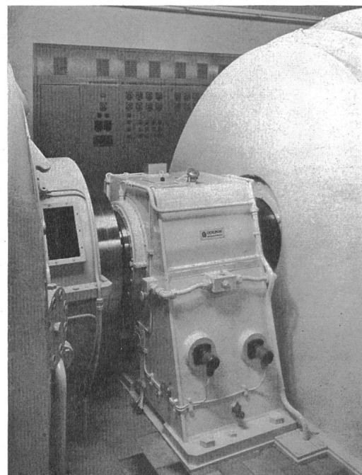
Fig. 10 Das Stehlager zwischen der Pumpe und dem Antriebsmotor
