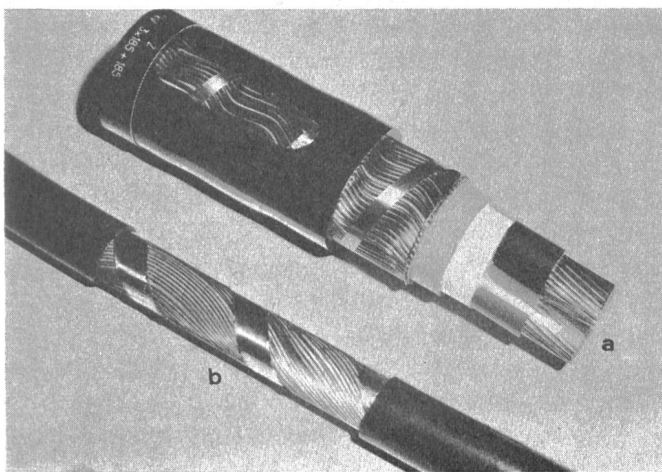
Fig. 6 Kabel mit konzentrischem Aussenleiter
