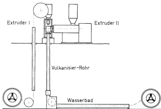
Fig. 12 CV-Vertikalanlage
