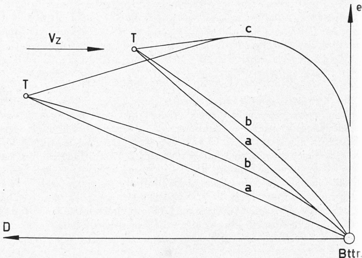
Fig. 1 Verschiedene mögliche Flugbahnen verhaltgelenkter Raketen auf den errechneten Treffpunkt T: a gerade Bahnen, b schnellste Bahnen, c Bahnen bei Senkrechtstart der Raketen.
