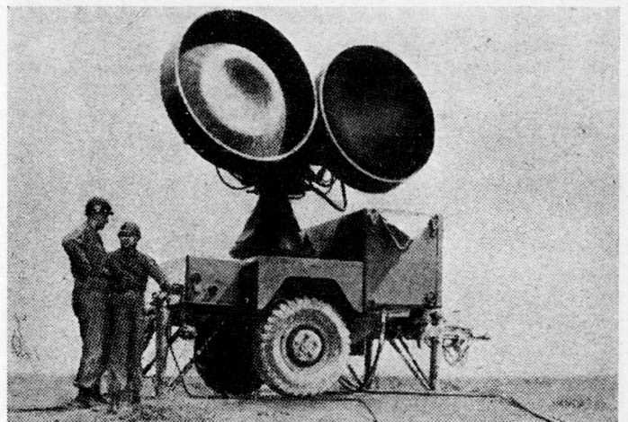
Bild 5. Beleuchtungs-Radar für die USA-Flab-Lenk Waffe «Hawk»
