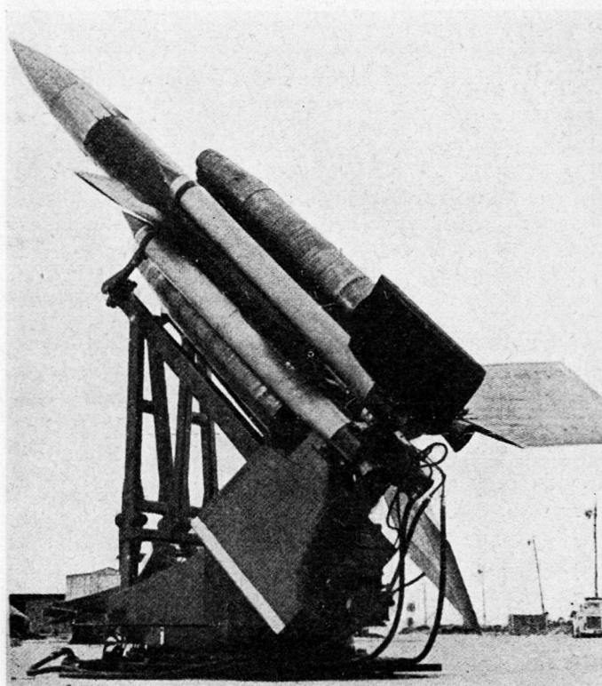
Bild 11. Startbereite Langstrecken-Flab-Lenk Waffe «Bloodhound» der britischen Luftwaffe
