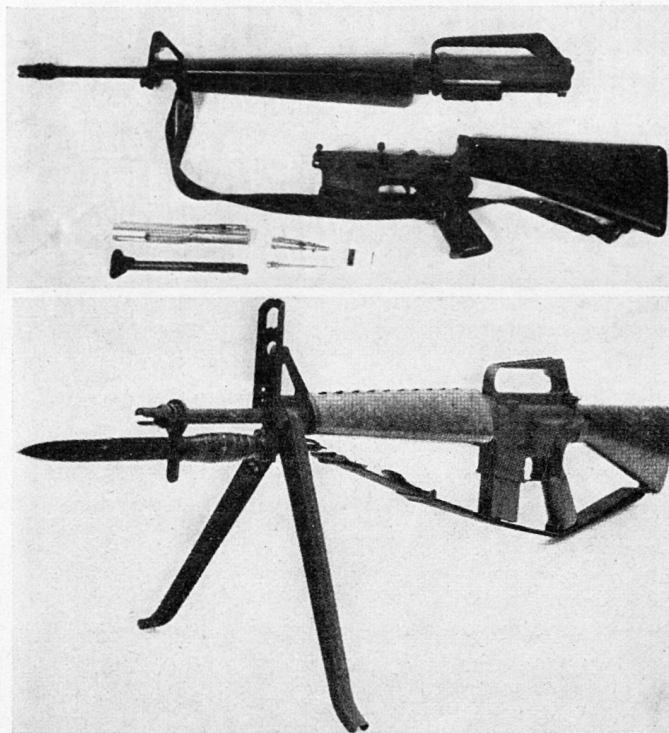
Das amerikanische Gewehr AR-15
