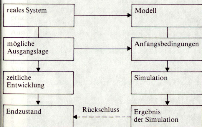
Beziehung Modell-Wirklichkeit
