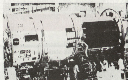
Die neue Orbitalstation «MIR» in der Montagehalle. Im Bild ganz rechts die Sektion mit den Kopplungssystemen. Telefotos: ZR/TASS
