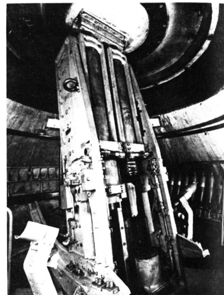
Bild 18. 12-cm-Festungsminenwerfer 59/83 (Geschützraum)
