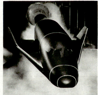
Modell des Raumgleiters «Her- mes» im Windkanal des Eidg. Flugzeugwerkes Emmen (Auf- nahme: F+W Foto- und Film- dienst)
