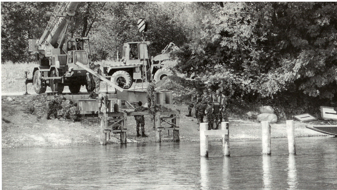
Abb. 4: Brückenbau mit Behelfsmaterial: Stahlträger werden auf gerammte Pfahljoche verlegt. (Versuchsstab Genie)
