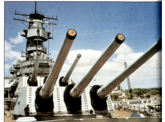
Abb. 3: Die 40,64-cm-Geschütze.
