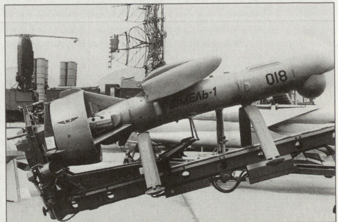
Aufklärungsflugkörper «Shmel-1» des russischen Drohnensystems «Malakhit».
