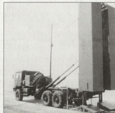
Prototyp eines leichten Abschussfahrzeuges für MEADS.
