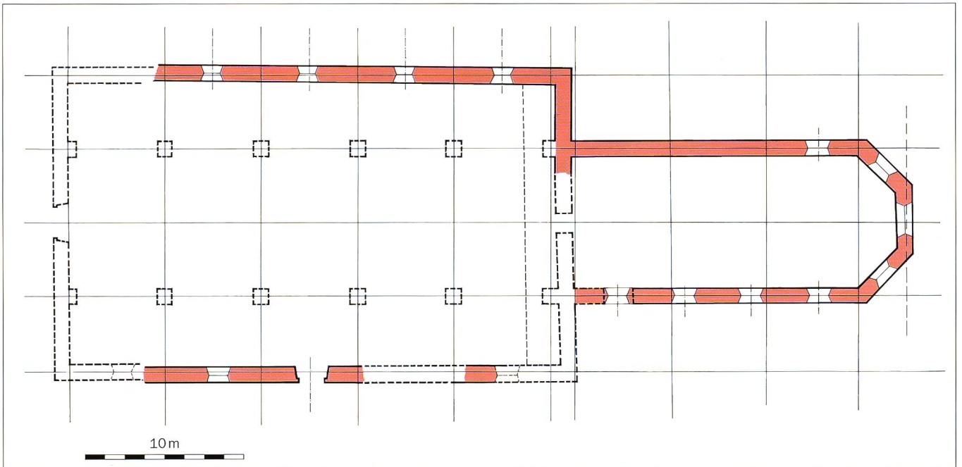
Abb. 55 Grundriss Gründungsbau, Rekonstruktionsversuch, 1:400. Eingefärbt = heute noch erhaltene Bauteile, Gestrichelte Linien = Rekonstruktion, Stichpunktete Linien = Fenster- und Türachsen, Feines Netz = Raster im Verhältnis 3:4 (Grundraster).
