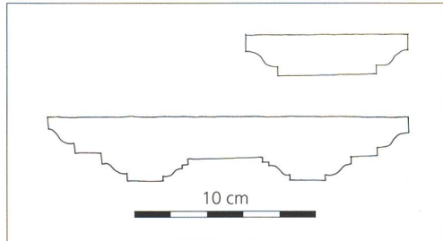
Abb. 12 Barfüßergasse 13, 3. Ober- geschoss, Täferdecke von 1641, Fundzustand, Profil Mittelfries und Deckleiste.
