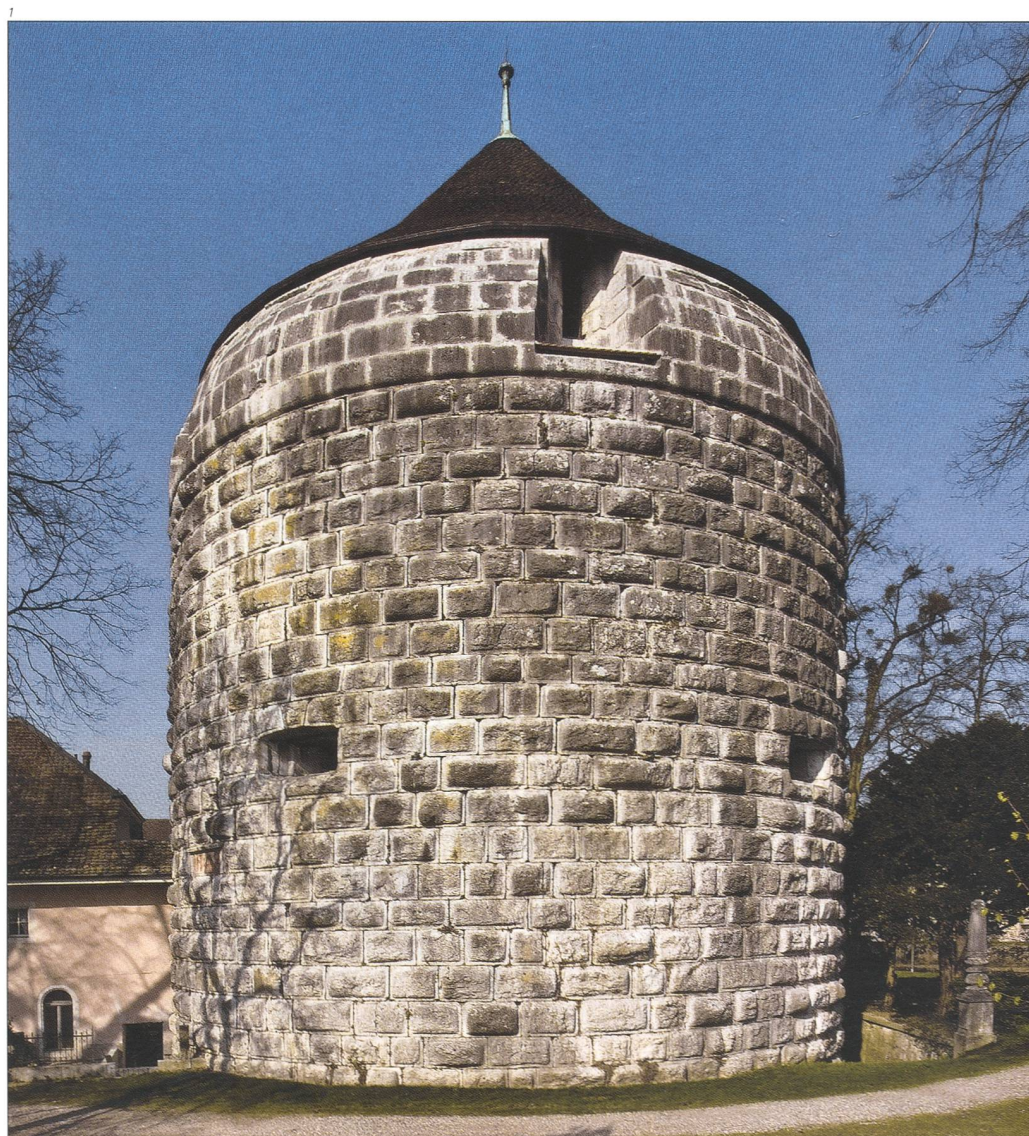
Abb. 1 Solothurn, Riedholzturm, Zustand Ostseite nach der Sanierung. Dachrinne und neue vermörtel- te Quaderfugen im abgerunde- ten Wehrgeschoss.
