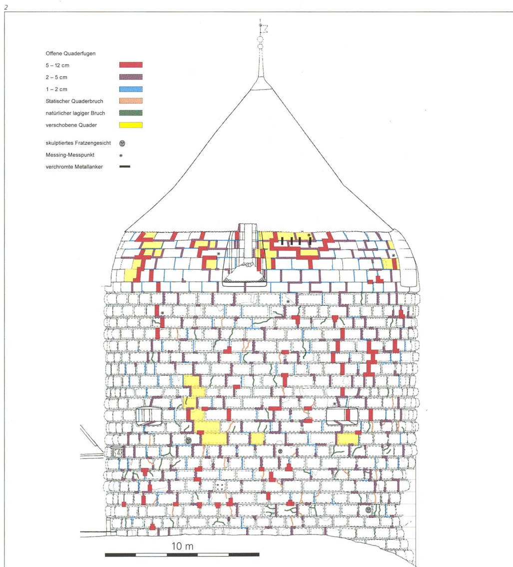
Abb. 2 Photogrammetrischer Aufnahmeplan der Ostseite. Schadenskartierung des Quadermauerwerks.
