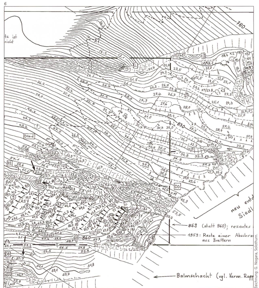
Abb. 6 Ausschnitt aus dem Handriss von Rudolf Glutz, Solothurn, der gemäss Definition sämtliche Messungen und Informationen enthält. Aufnahme im Massstab 1:500, abgebildet im Massstab 1:1000.
