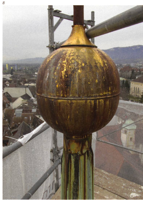
Abb. 8–13 Zustand des Kupferblechs von 1925 mit korrodierten Stellen, Ausbesserungen aus verschie- denen Zeiten, Rissen im Blech, Schäden an der Kugelvergold- ung und verrosteter Wetter- fahne. Foto 2015.
