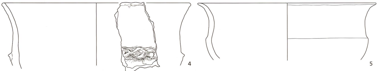
Taf. 1 Keramik. 1–5 Schüsseln. M 1:2.
