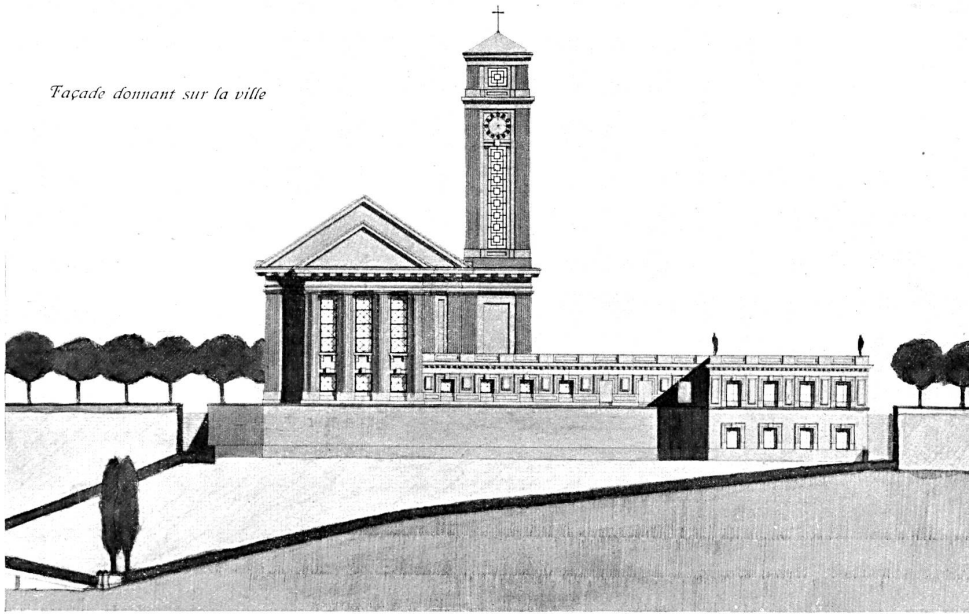
Concours pour l'érection de l'église réformée de Fluntern à Zurich. Projet de l'architecte Paul Vollenweider, Zurich.
