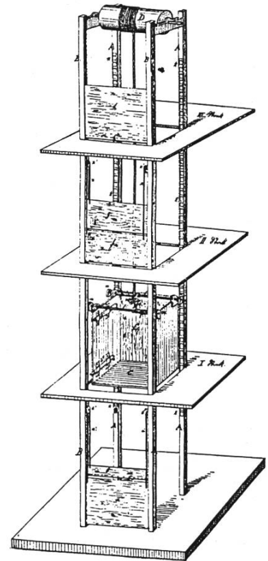
Bild 2. Fahrstuhlmodell mit Schutzvorrichtung, System Nüesperli
