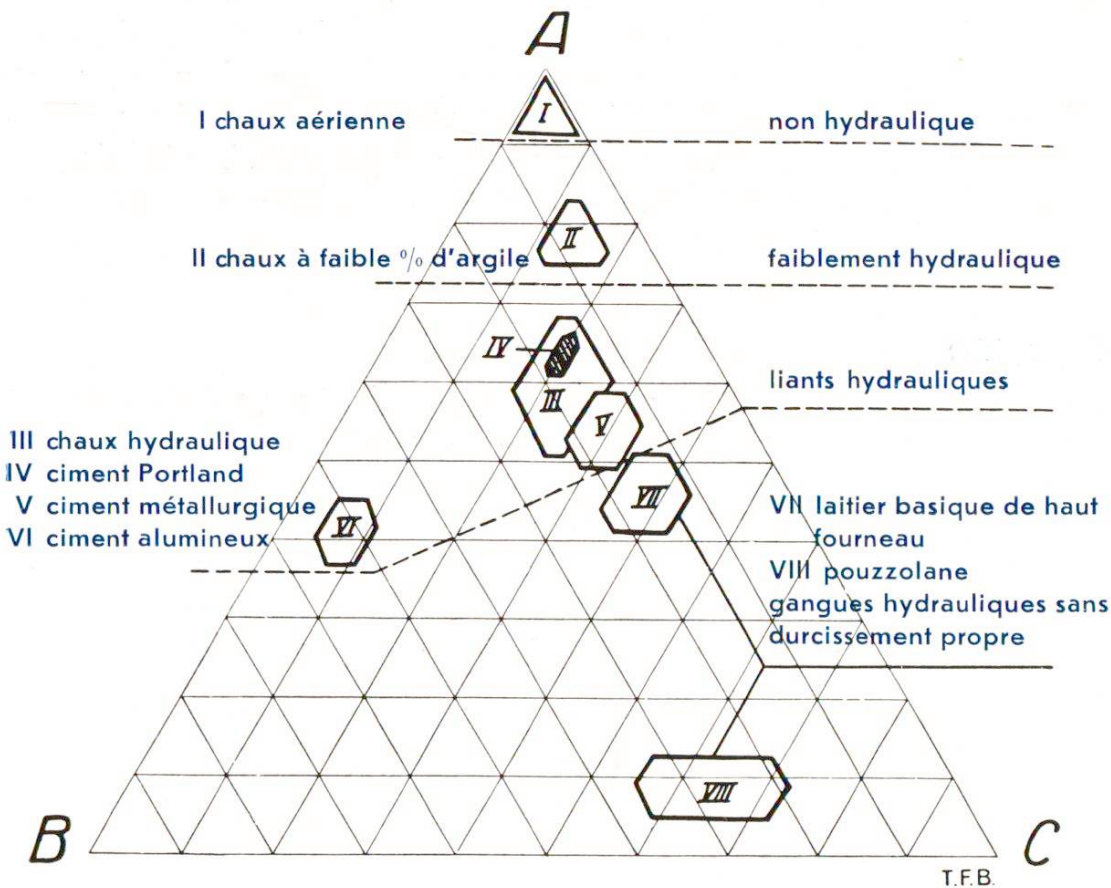
Fig. 2 Les liants dans le système ternaire. Diagramme triangulaire avec la chaux (A=100%), l'alumine (B=100%) et la silice (C=100%)
