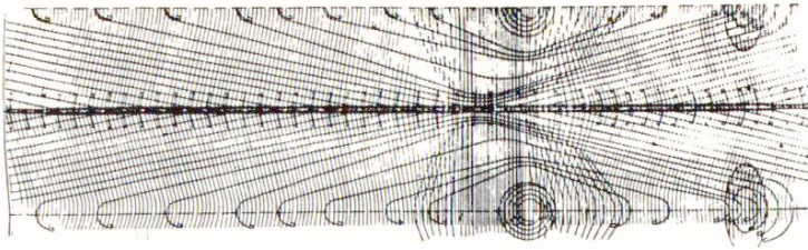
Fig. 3 Tribunes du champ de course à Madrid. En bas: coupe transversale de la construction en béton armé. En haut: armature des voiles minces
