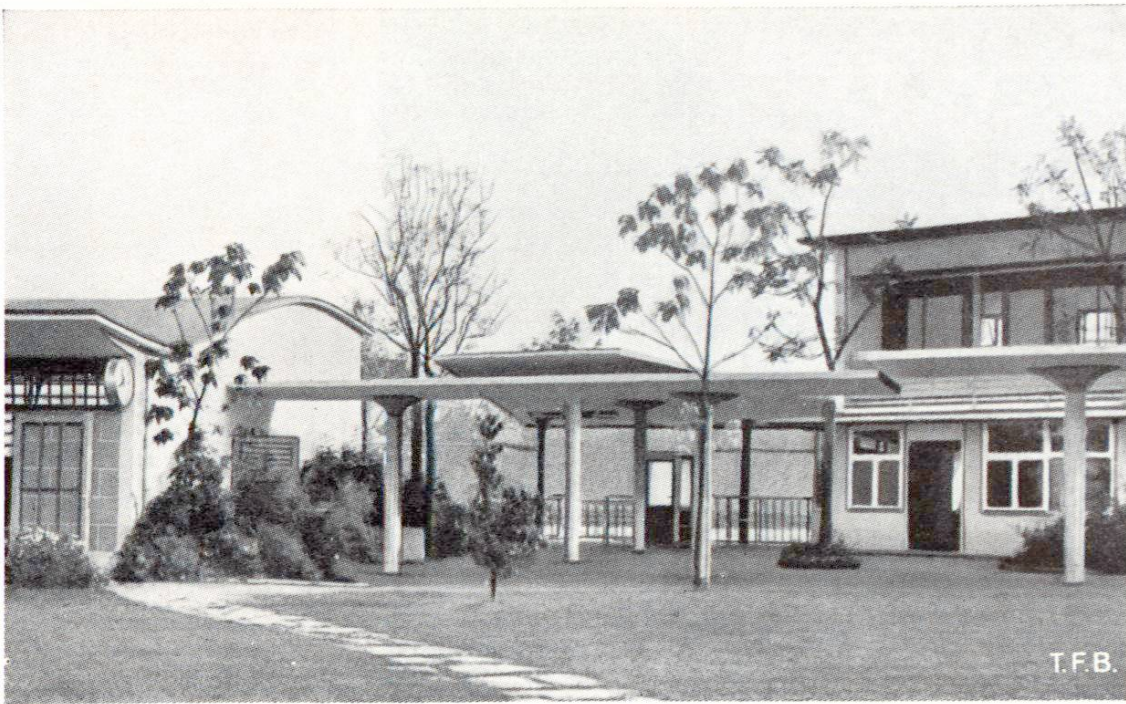
Fig. 7 Entrée des bains à ciel ouvert d'Allenmoos, à Zurich. Constructions brutes en béton armé. Toits-champignons isolés pour les passages couverts. A gauche, vestiaires à toit élargi en béton armé
