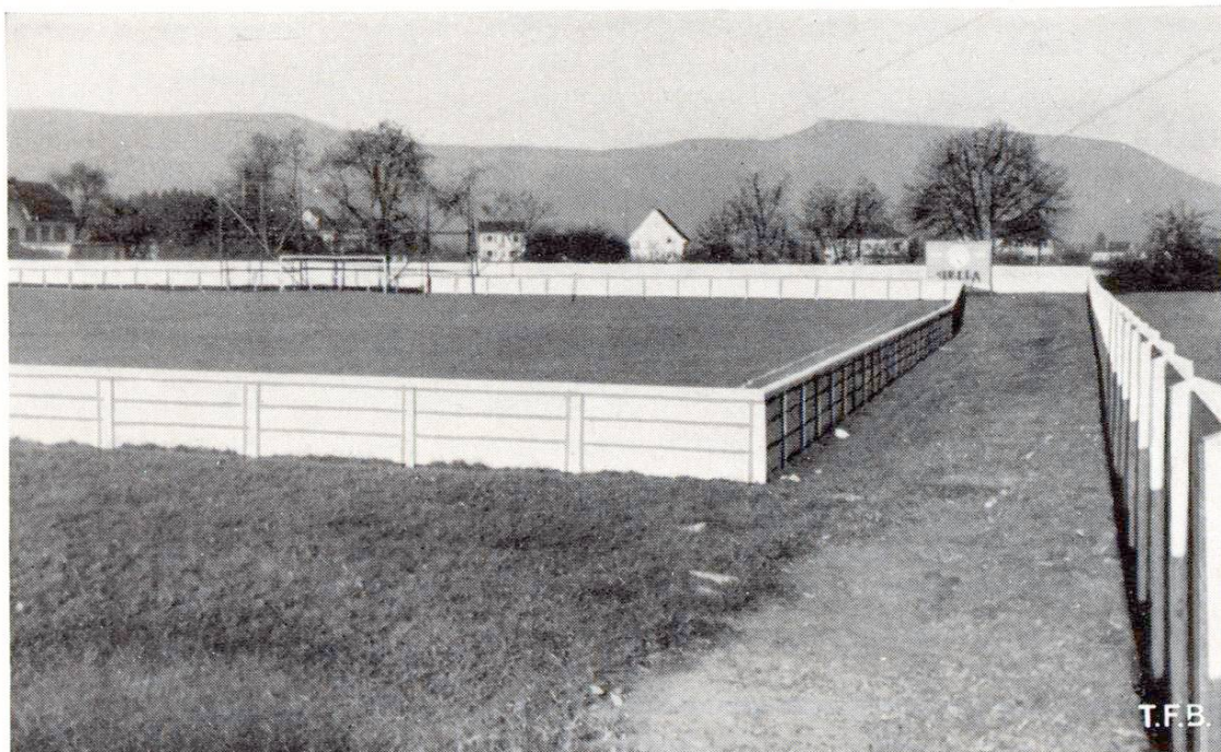
Fig. 4 Clôtures de la place de sport Brüggelfeld, à Aarau. Éléments en béton préfabriqués
