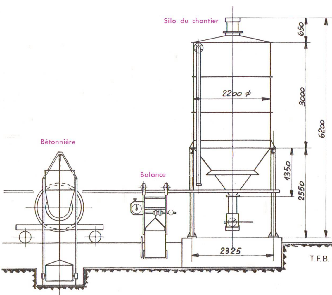
Fig. 8 Installation du chantier pour ciment en vrac. Silo de 15 t
