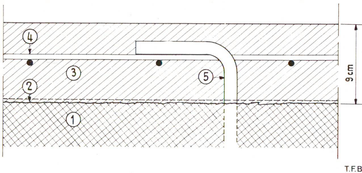
Fig. 1 Revêtement mince. 1 = Béton de construction, 2 = Surface rugueuse, enduite de mortier, 3 = Béton de revêtement BH 350, 4 = Treillis d'acier, 5 = Fers de liaison
