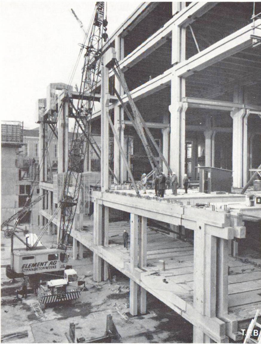
Fig. 8 Vue du montage d'une travée. Il fallut chaque fois 10 jours de travail pour monter les 5 étages d'un axe (277 éléments).
