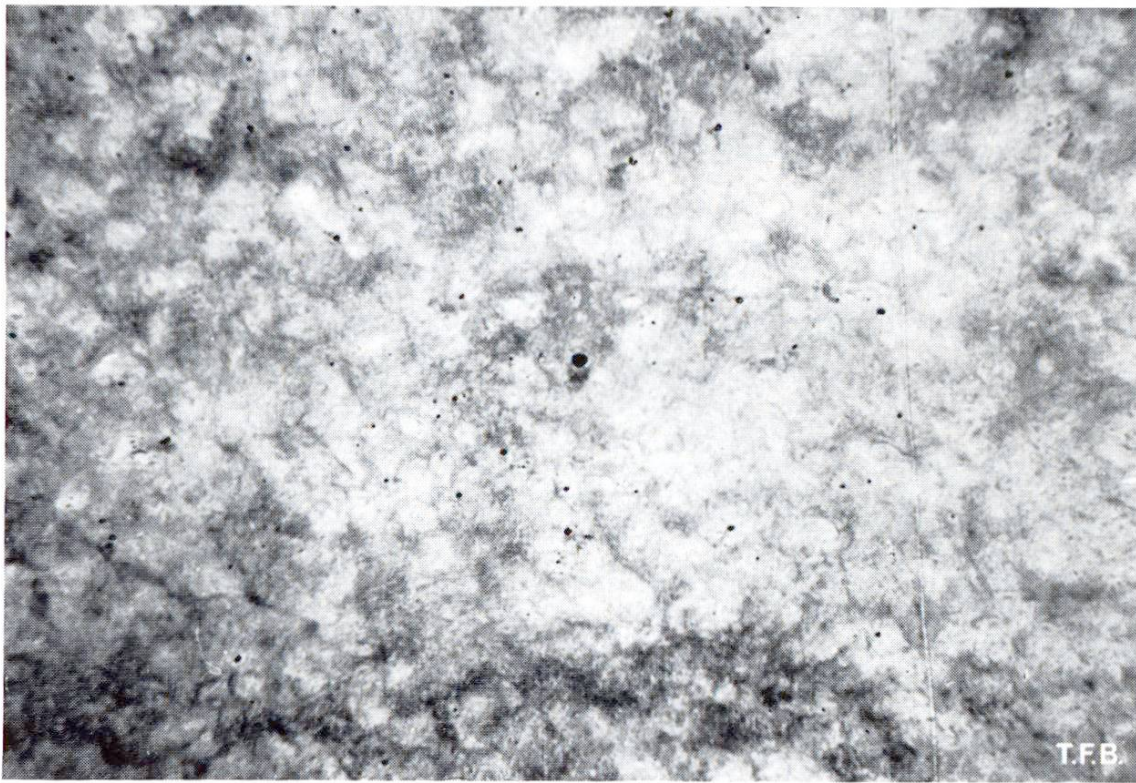
Fig. 5 Séparation entre eau et ciment aux endroits où les gros grains sont en contact avec le coffrage. Les granulats transparissent. On peut éviter cela en augmentant la durée du malaxage.
