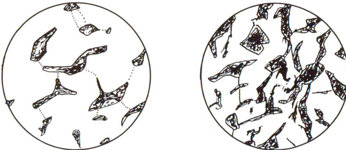
Fig. 1 Représentation schématique des pores de la pâte de ciment (diamètre du dessin env. 0.005 mm). A gauche: e/c 0.45, teneur en pores capillaires env. 10 %. Les vides ne sont reliés entre eux que par les pores du gel (en pointillé). A droite: e/c 0.8, teneur en pores capillaires env. 40 %. Les vides forment un réseau continu.
