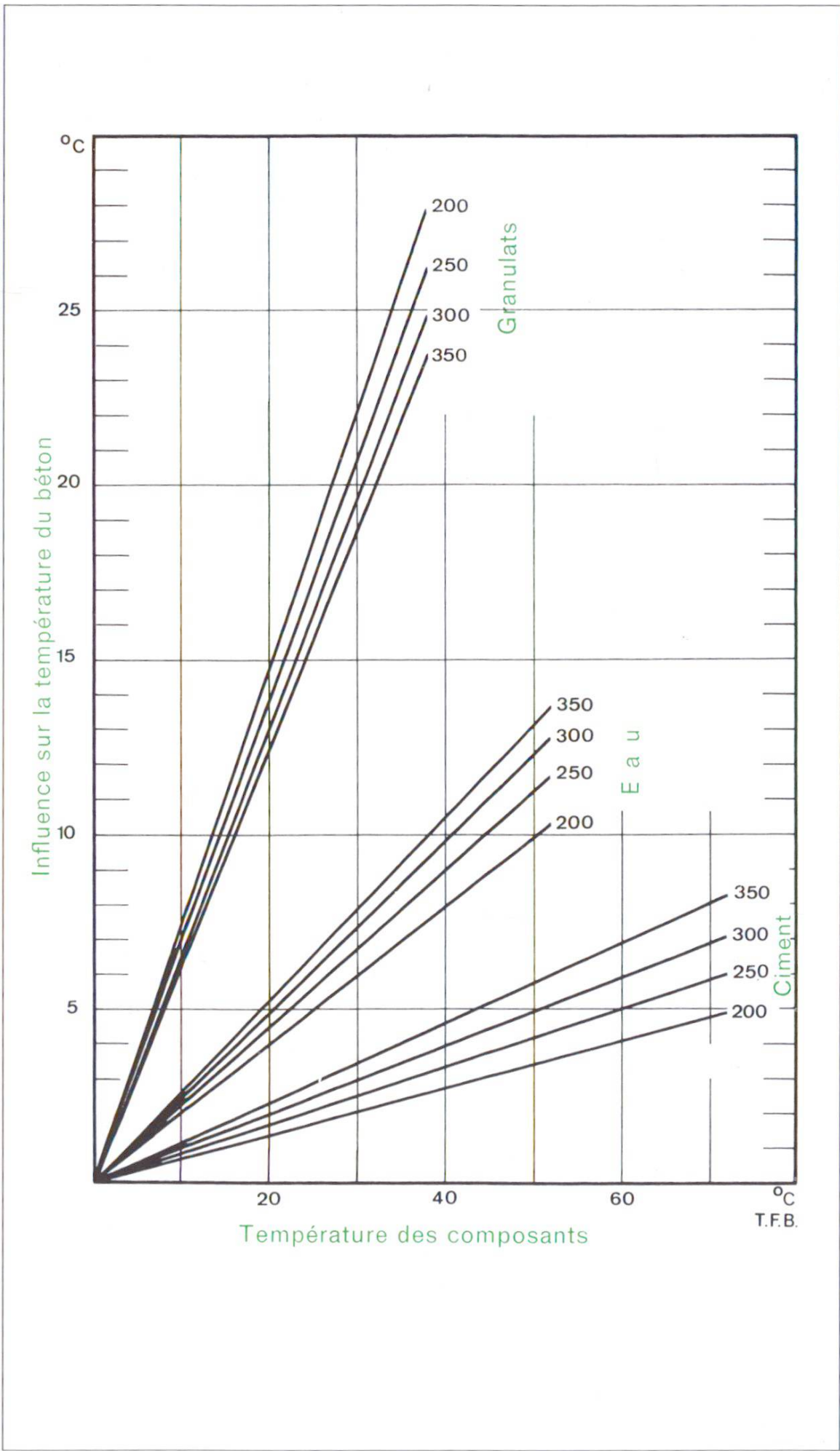
Fig. 1 Diagramme permettant de déterminer la température du béton frais à partir de celles des granulats, du ciment et de l'eau de gâchage, pour des dosages en ciment de 200, 250, 300 et 350 kg/m³. La somme des températures lues en ordonnée donne celle du béton frais.
