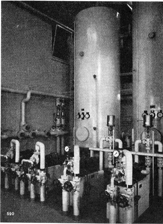
Sulzer Heizungs- und Verteilzentrale mit Brauchwasser-Speicheranlage
