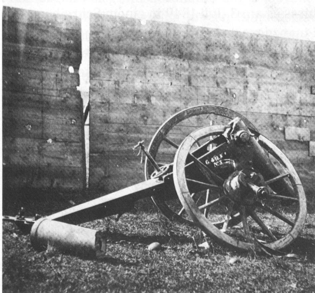
Zersprungenes Kanonenrohr als Folge der vom Bund gelieferten unpassenden Pulverqualität. (Quelle: Brunisholz, Pulver, 191)
