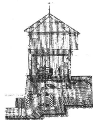
Querschnitt durch das Maschinenhaus.
