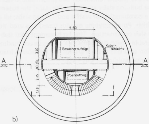
Schaft, Aufzugschächte und Treppenanlage a) Ansicht und Schnitt A - A b) Horizontalschnitt
