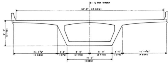
Fig. 2 Transverse section
