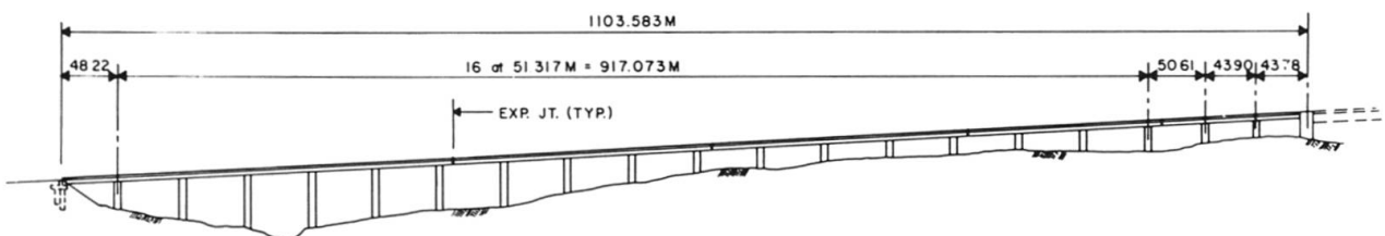
Fig. 1 Elevation
