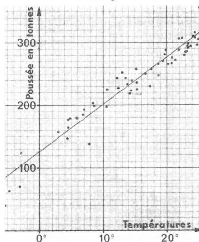
Fig.14 - Relation poussée-température
