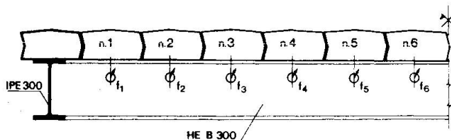
Fig.1 - Disposition d'essai
