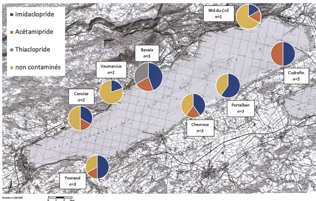
Figure 5. Carte des contaminations par zone de pêche. Les graphiques à secteurs représentent la proportion de contamination par l'imidaclopride, l'acétamipride et le thiachlopride. Les secteurs sont calculés en proportion du nombre total de contaminations. Exemple: Une moule contaminée par deux néonicotinoïdes différents est comptée comme deux contaminations. n représente le nombre d'individus contaminés par au moins un néonicotinoïde. Carte du lac de Neuchâtel prise sur le site du SITN : https://sitn.ne.ch/theme/main
