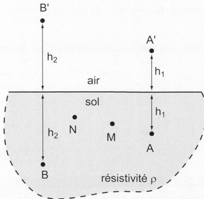
Figure 3.—Le quadripôle électrique de mesure. Comme les électrodes d'injection de courant A et B se trouvent sous la surface du sol, il est nécessaire de tenir compte des images de ces électrodes ( A' et B' ) lors du calcul du facteur géométrique G .
