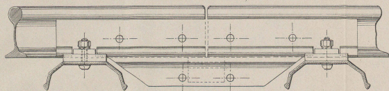
Fig. 10 Eclisse à pont.
