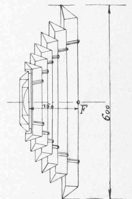
Profil d'optique lenticulaire.
