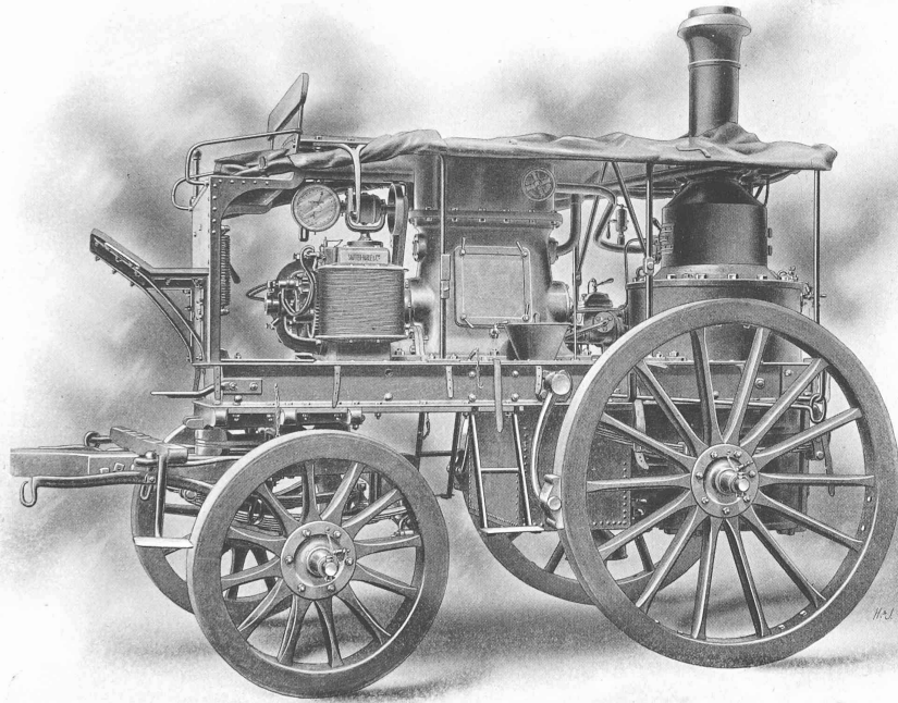
LOCOMOBILE A LUMIÈRE POUR USAGES MILITAIRES (SAUTTER, HARLÉ & C ie )
