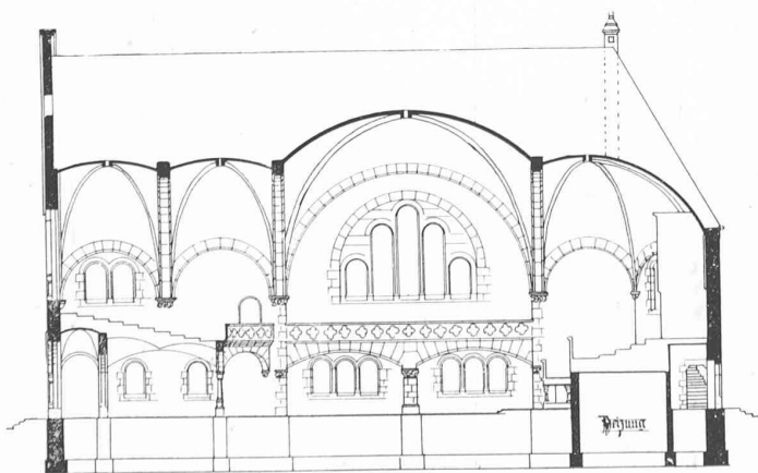
COUPE LONGITUDINALE (1 : 500)
