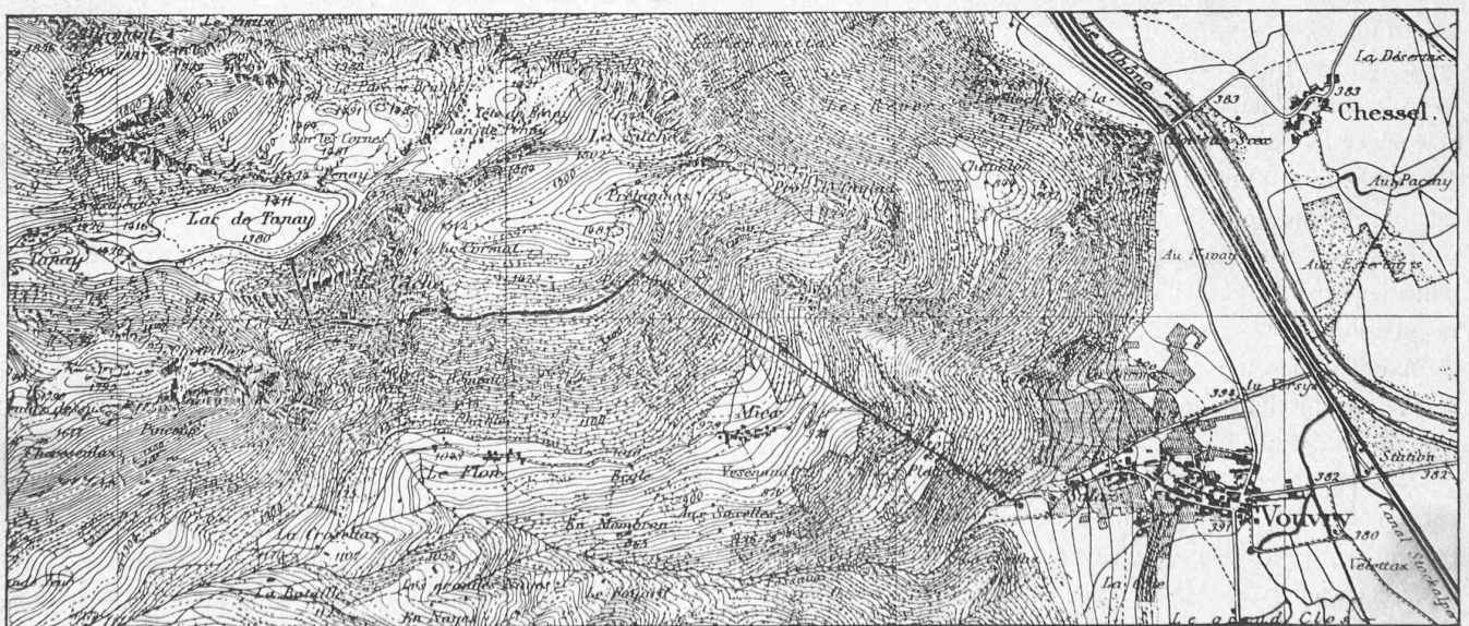
Fig. 3. — Plan général de l'installation.
