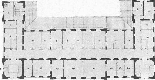
Fig. 8. — Plan du 1 er étage.
