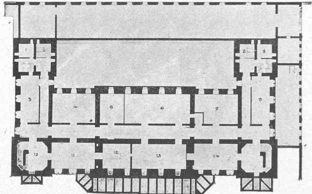
Fig. 9. — Plan du sous-sol.
