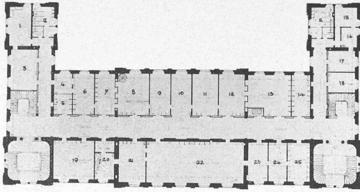
Fig. 6. — Plan du 2 me étage.
