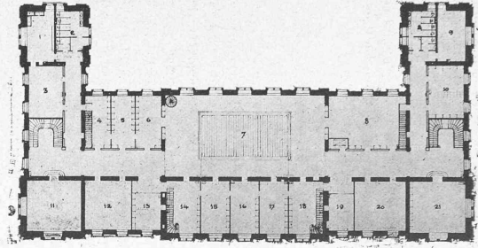
Fig. 7. — Plan du 3 me étage.
