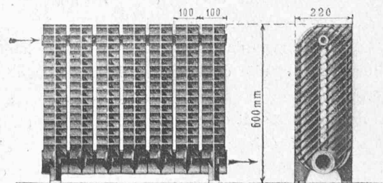
Fig. 19. — Radiateur à ailettes.
