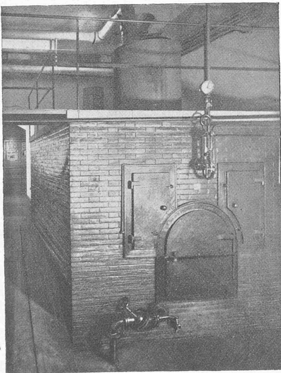
Fig. 16. — Chaudière.
