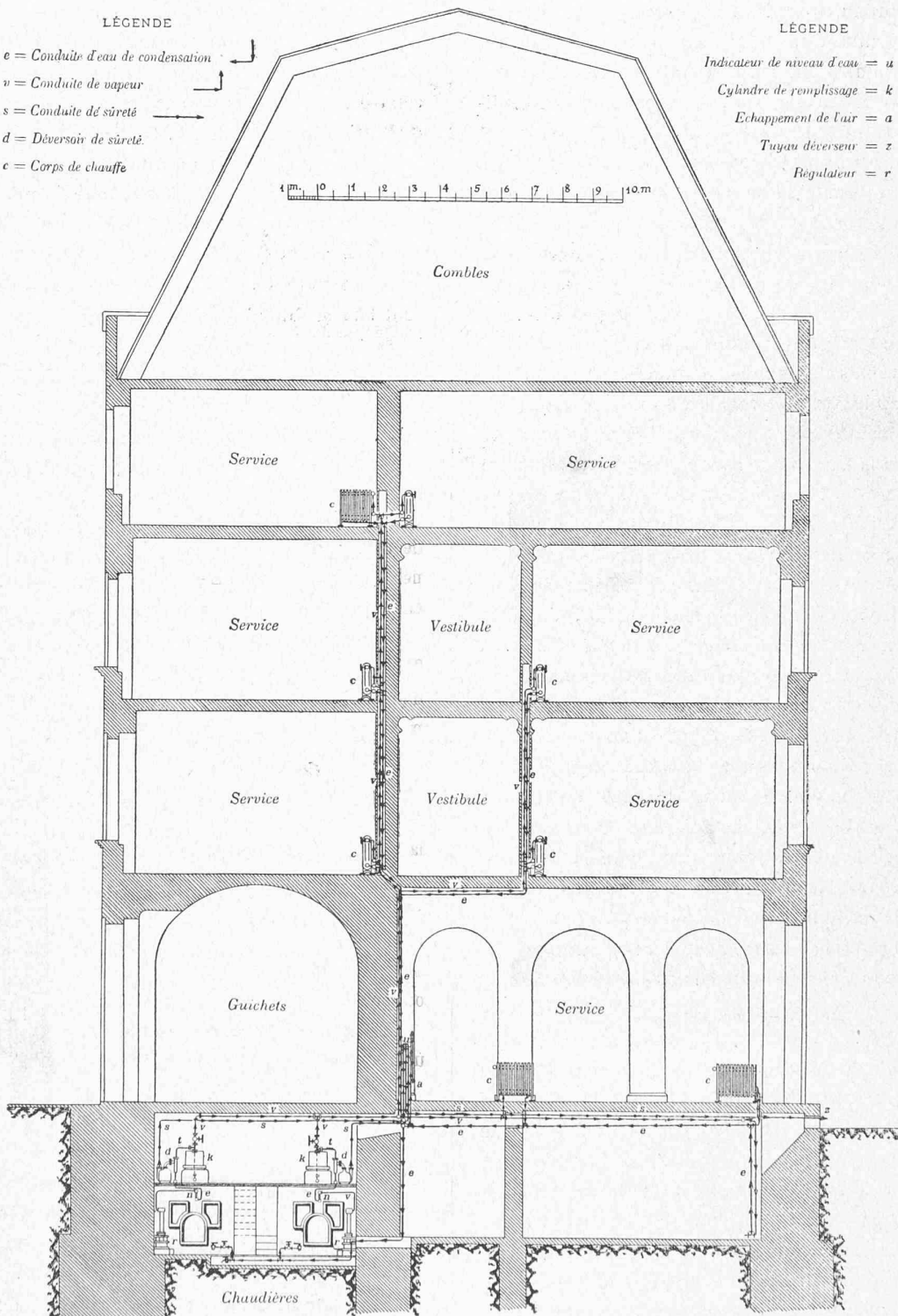
HOTEL DES POSTES DE LAUSANNE - CHAUFFAGE CENTRAL A VAPEUR INSTALLÉ PAR MM. SULZER FRÈRES, A WINTERTHUR
