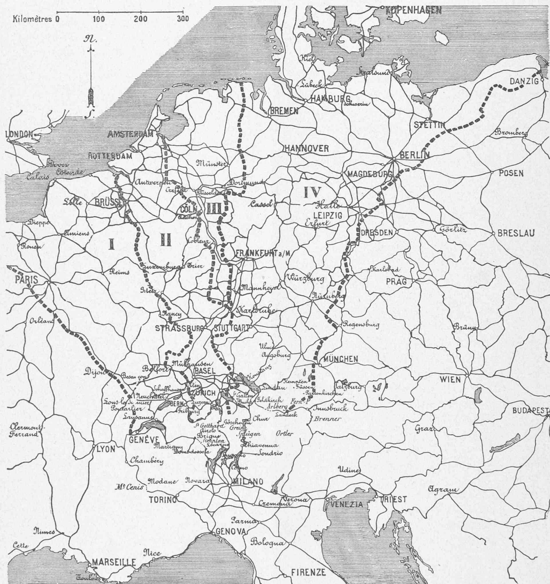
Fig. 1. — Carte des zones de trafic des lignes de chemins de fer construites ou projetées à travers les Alpes suisses, le trafic italien étant supposé concentré en un point situé près de Crémone.
