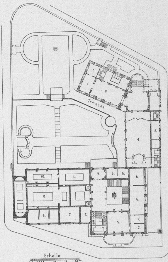
Fig. 11. — II m e Prix « ex æquo » : Projet n° 23 « Kunstgütterli ». Plan de l'étage principal.
