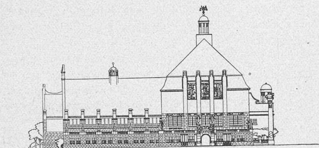
Fig. 9. — II m e Prix « ex æquo » : Projet n° 23 « Kunstgütterli ». M. KARL MOSER, de Baden (Argovie), architecte, à Karlsruhe. Façade sur la place Heim.
