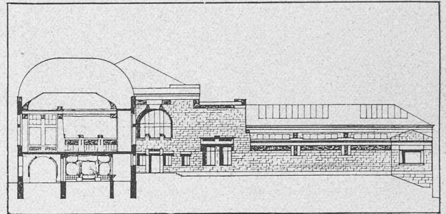
Fig. 7. — II me Prix « ex æquo »: Projet n° 22 « Stein und Bronze ». Coupe et façade sur le jardin.
