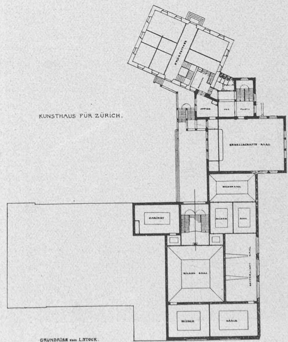
Fig. 8. — II me Prix « ex æquo »: Projet n° 22 « Stein und Bronze ». Plan du premier étage.
