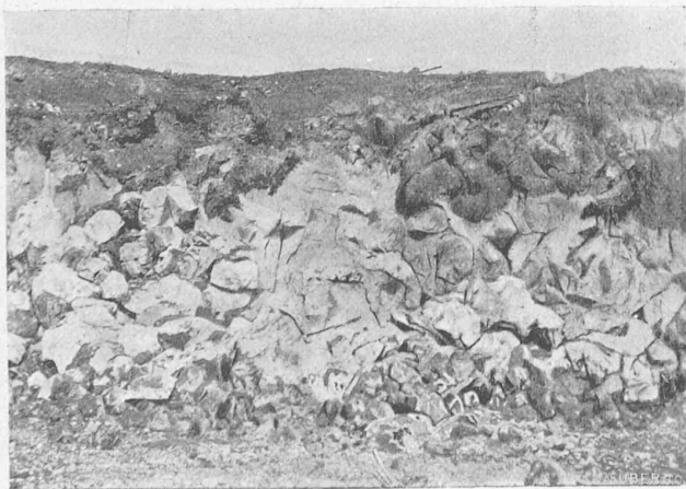
Fig. 3. — Massif éboulé.
