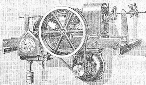
Treuil élévateur pour monte-plats. Système Binkert.
